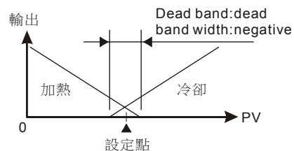
圖六：PID控制，Dead band為負值
