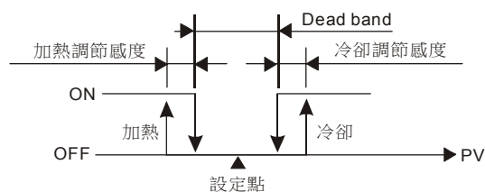
圖四：雙輸出ON-OFF控制時輸出運行圖示
